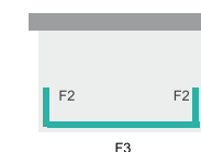
Sprchovací kút - kombinácia pevných skiel OASIS F2 + F3 + F2
