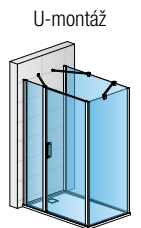
U-montáž D22T31 + D22F1 + D22F3 + D22EV1.10.500 + D22EV2.10.500
